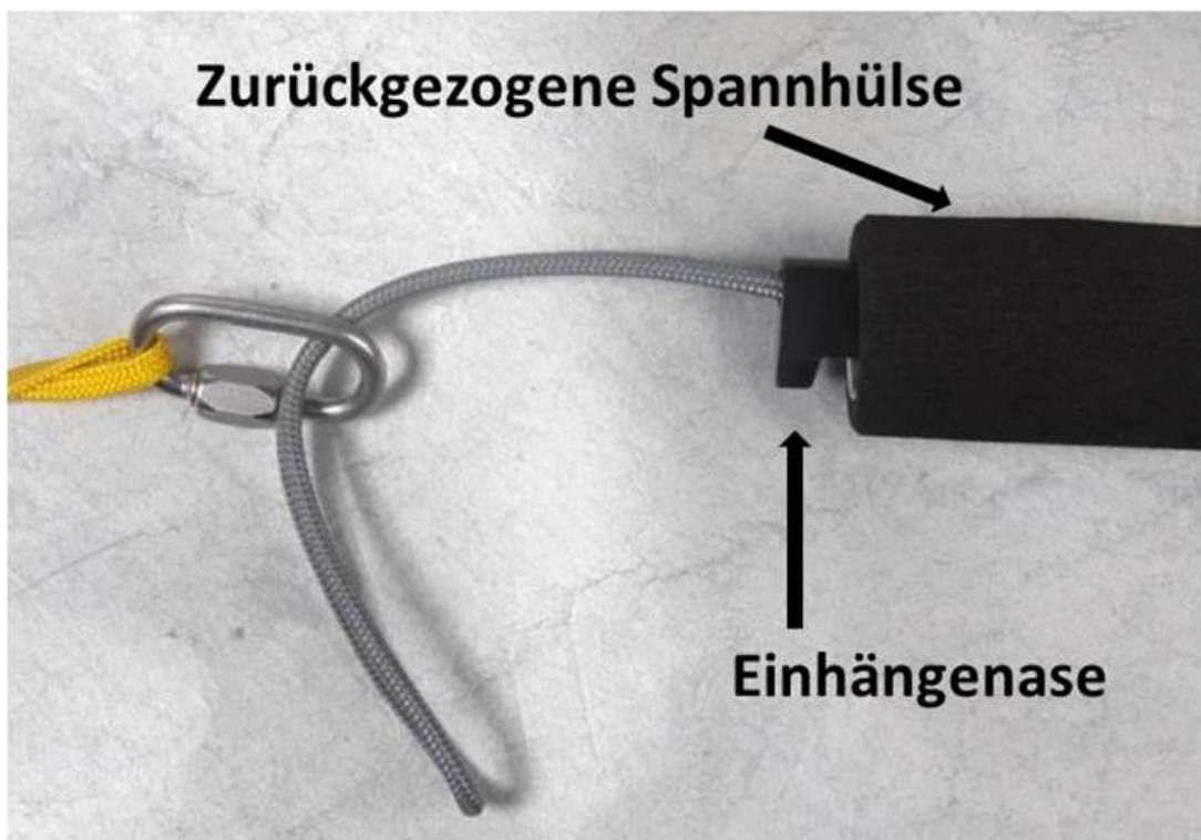
Abbildung 5.1: Spannhülse zurückgezogen
