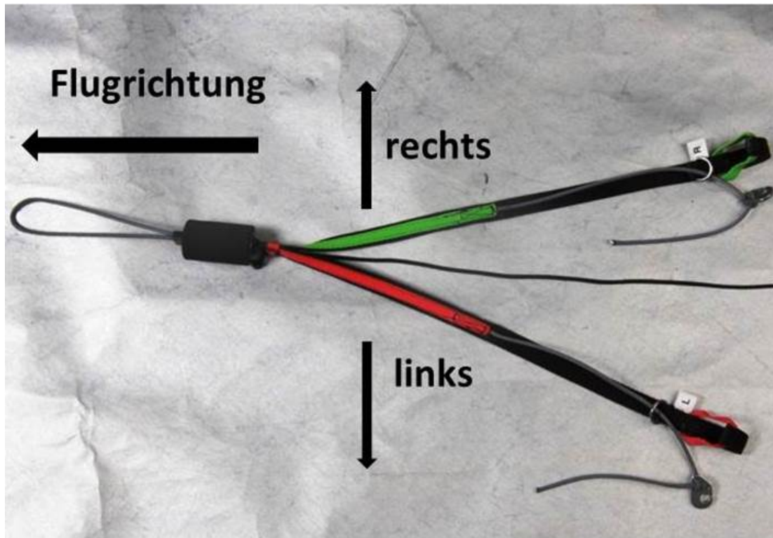
Abbildung 4.2: Farbliche Markierung der Schleppklinke (Draufsicht)
